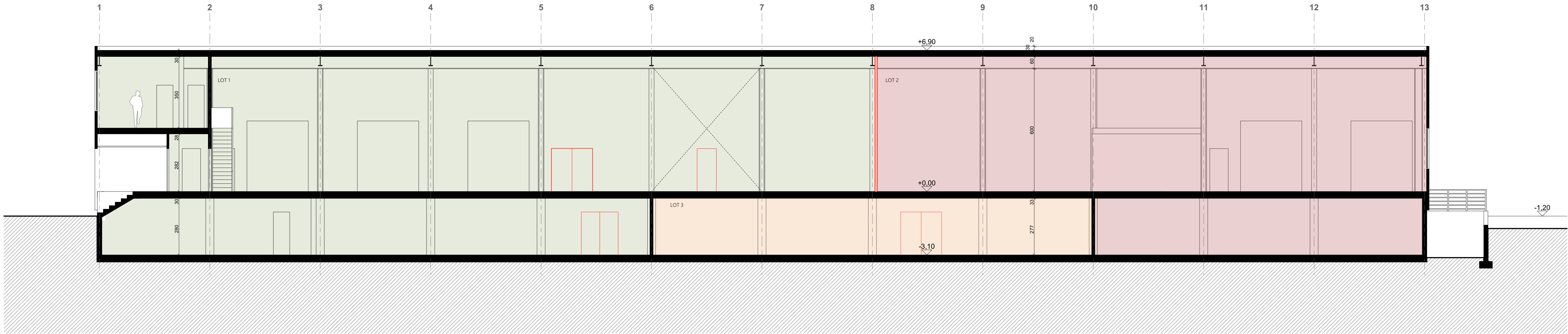
Coupe B-B 1/100
