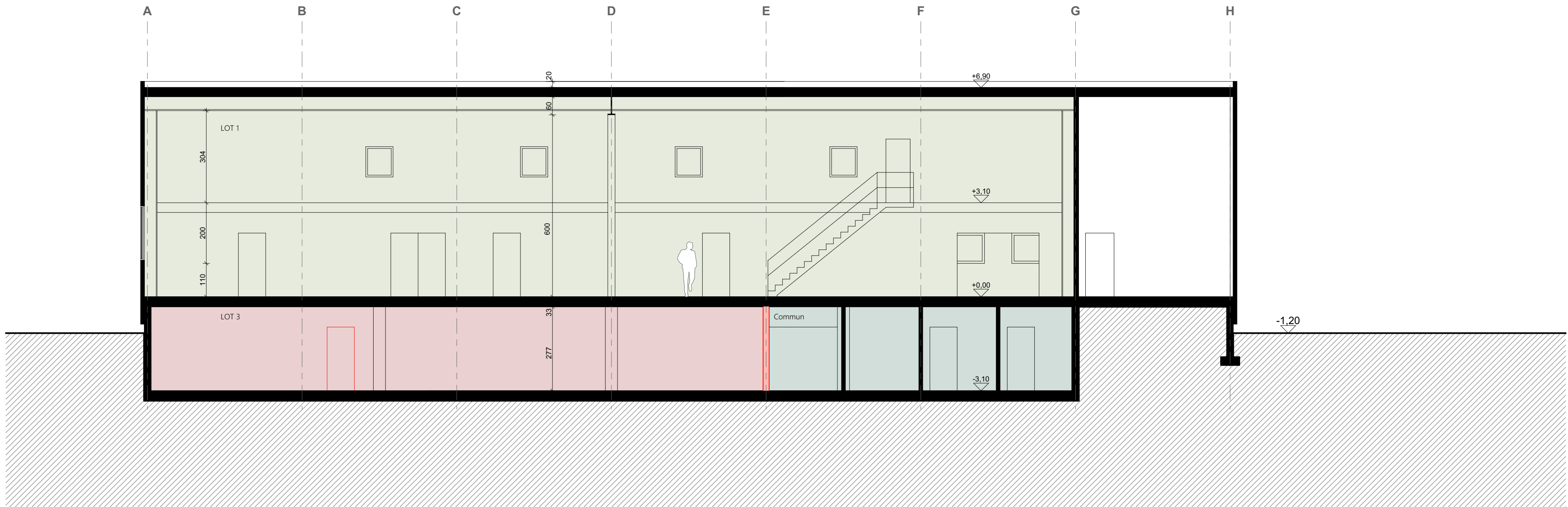
Coupe A-A 1/100
