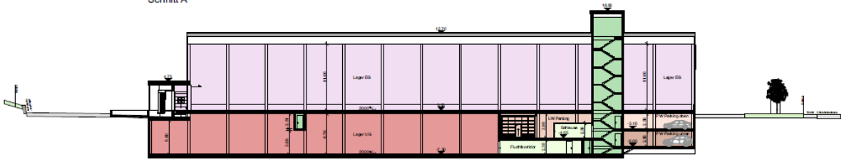
Schnitt A
